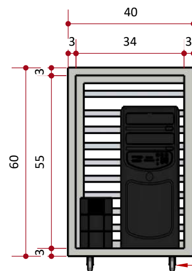
VISTA FRONTAL MÓVEL P/ GABINETE
