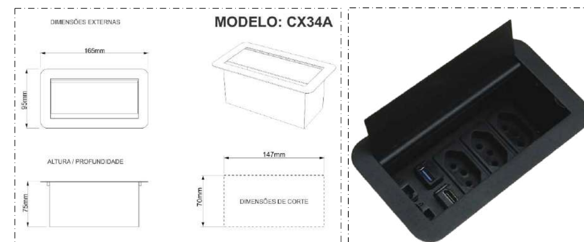
CAIXA TOMADA
