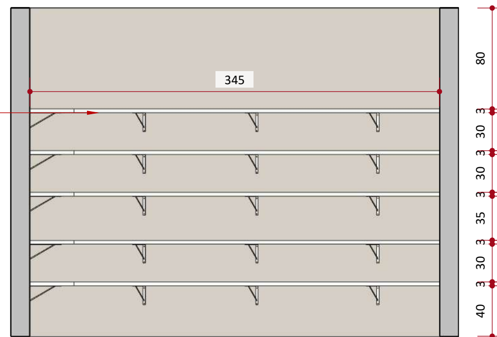
Vista 7 - Despensa ESCALA 1:30
