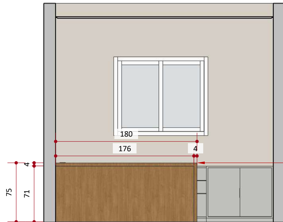
Vista 4 ESCALA 1:30
