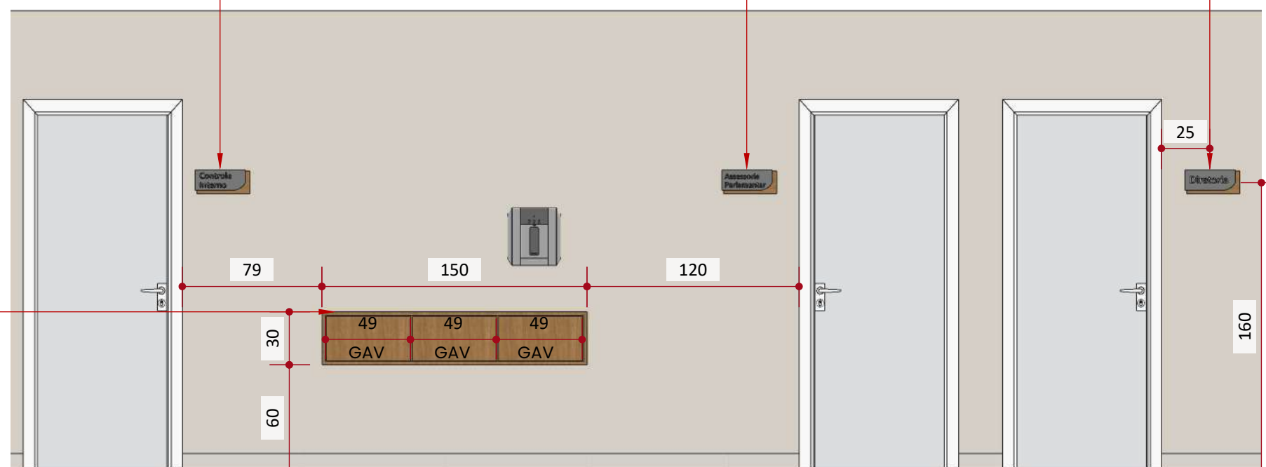
Vista 2 ESCALA 1:30
