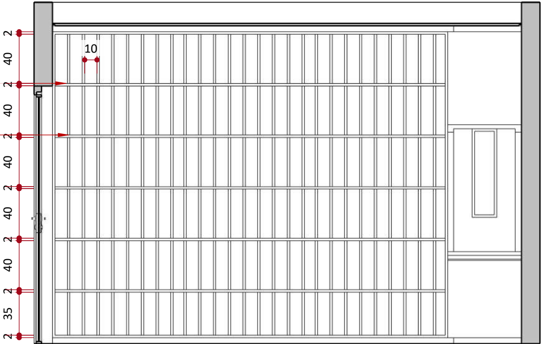
Vista 02 - Interno ESCALA 1:30
