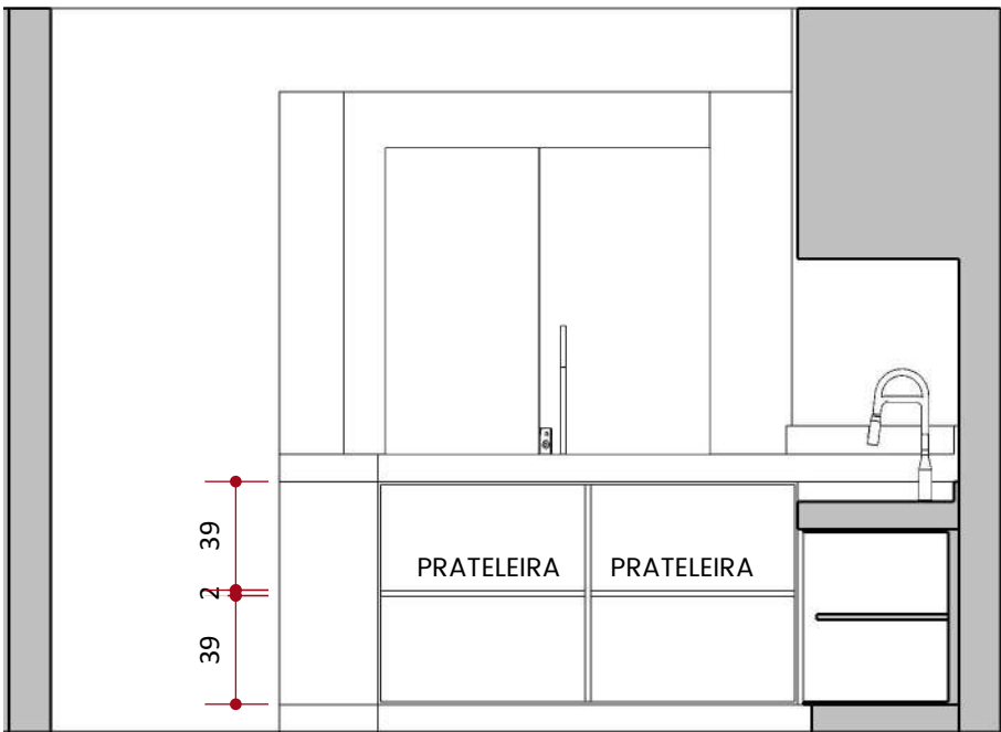
Vista 08 - Cozinha ESCALA 1:30
