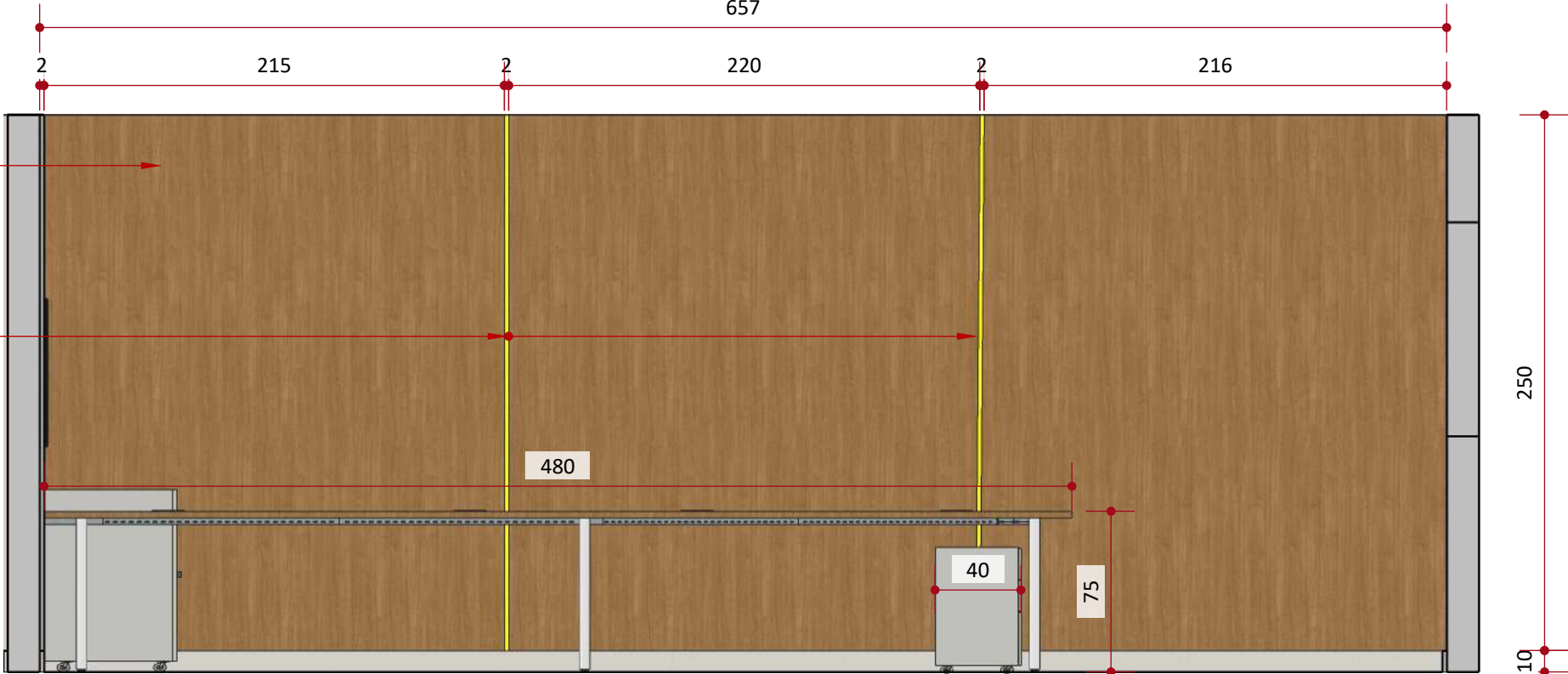
Vista 3 - Sala do presidente ESCALA 1:30
