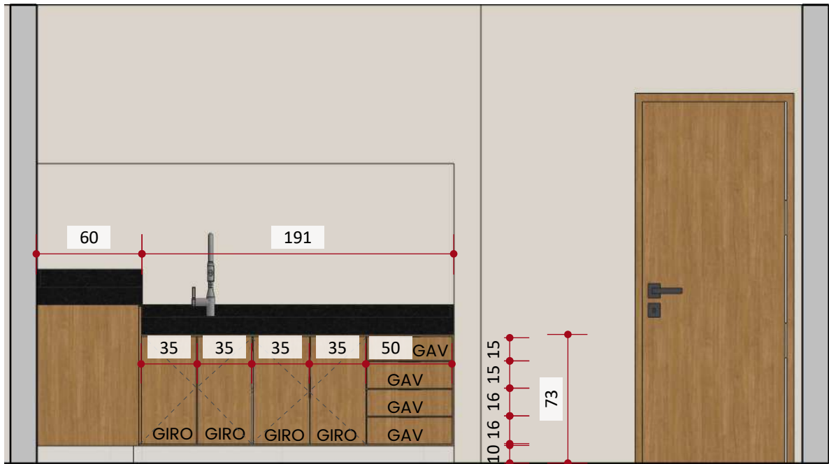
Vista 9 - Cozinha ESCALA 1:30
