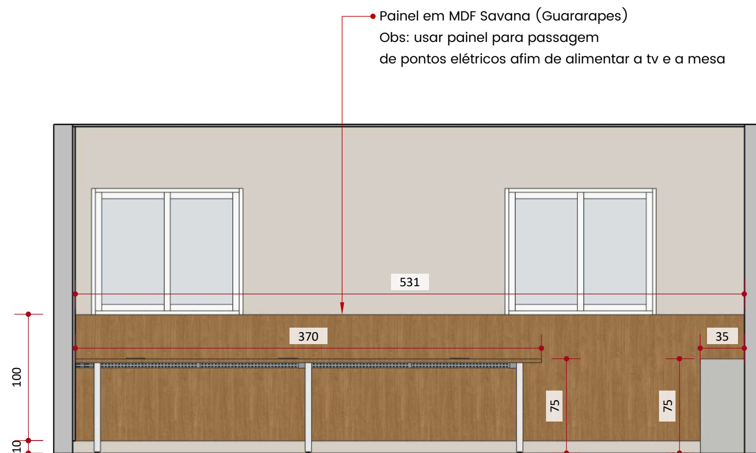
Vista 3 ESCALA 1:30
