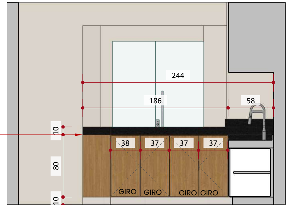
Vista 8 - Cozinha ESCALA 1:30
