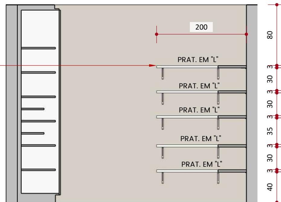
Vista 6 - Despensa ESCALA 1:30
