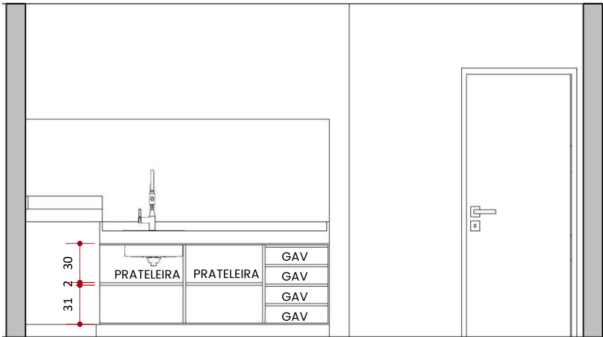
Vista 09 - Cozinha ESCALA 1:30
