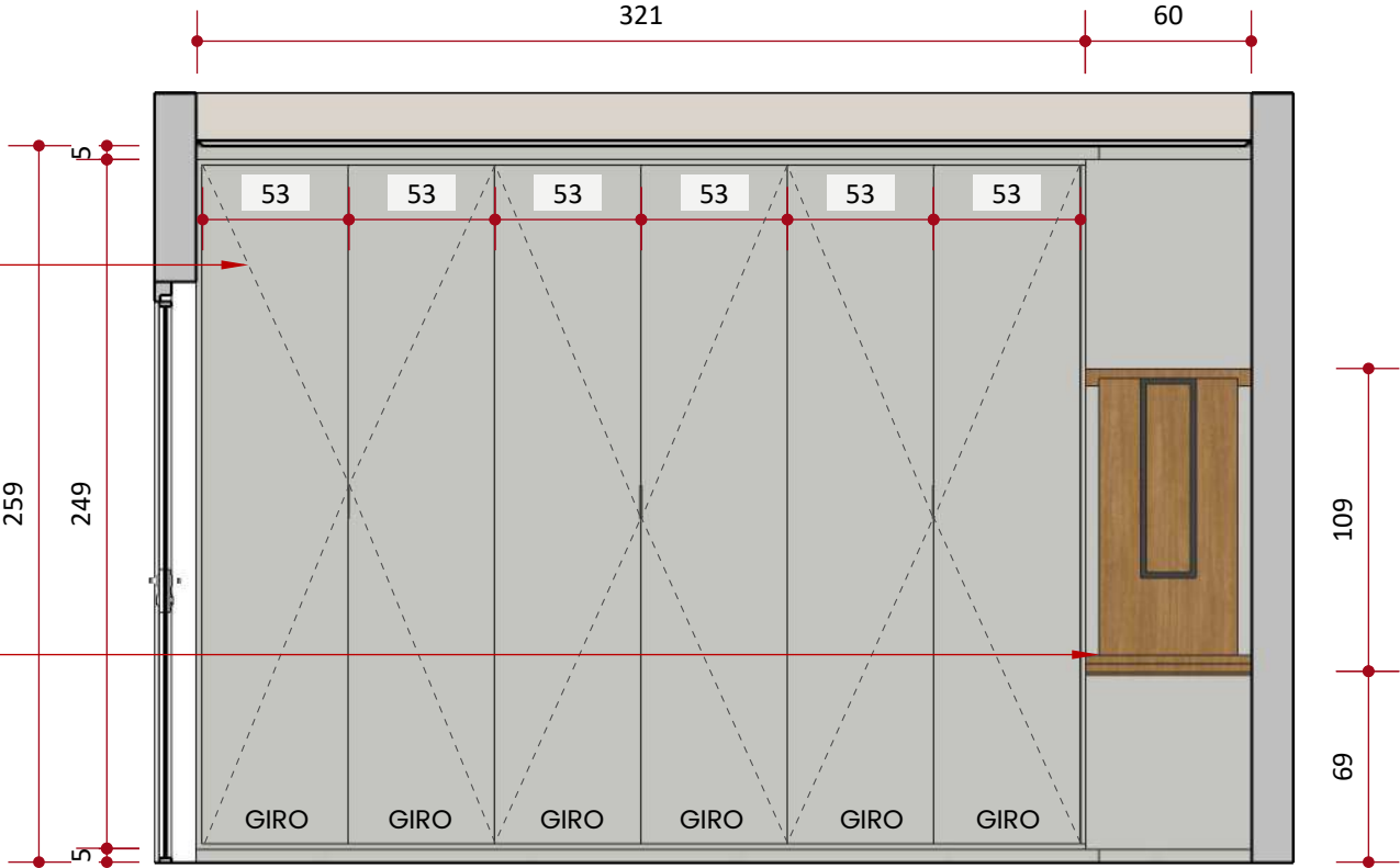
Vista 2 ESCALA 1:30
