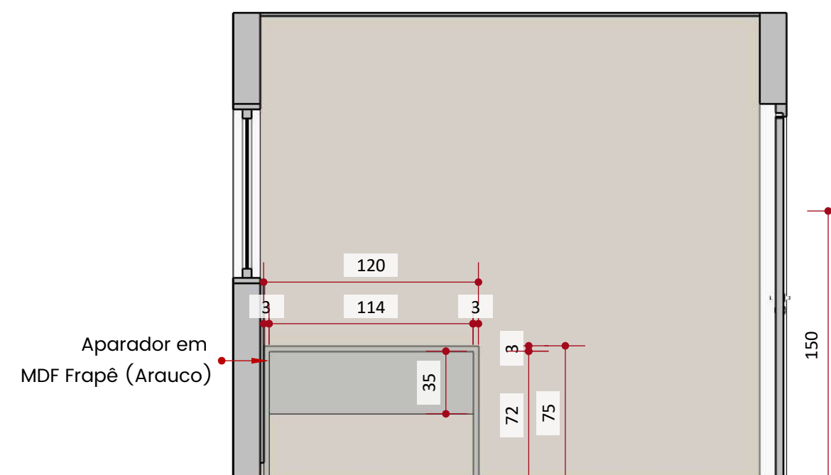
Vista 4 ESCALA 1:30
