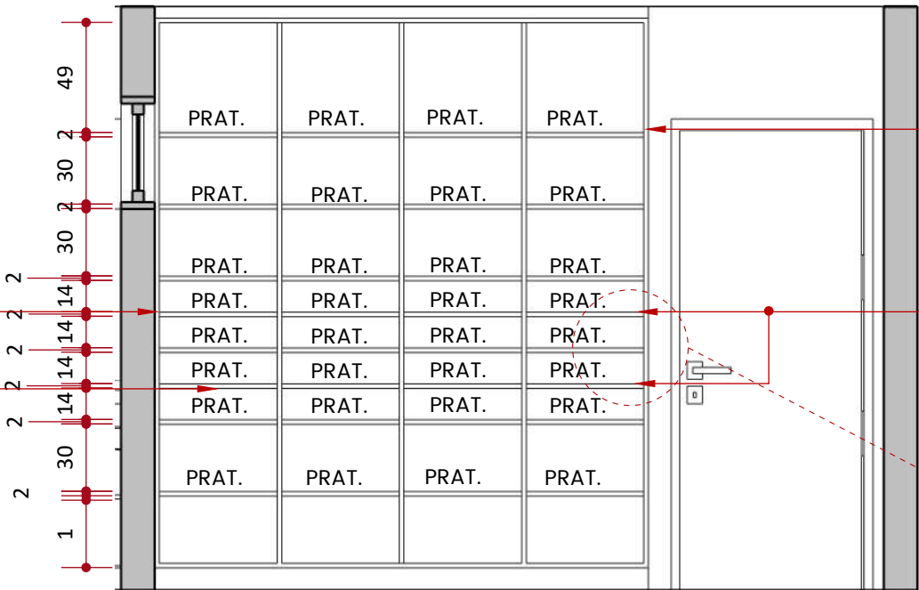
Vista 05 - Interno ESCALA 1:30
