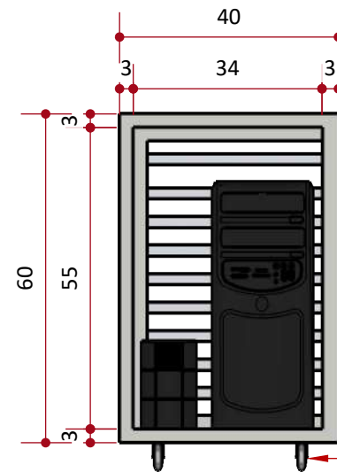
VISTA FRONTAL MÓVEL P/ GABINETE
