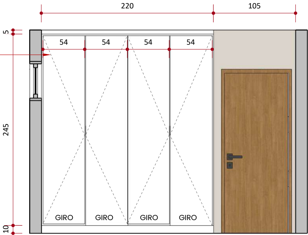
Vista 5 - Despensa ESCALA 1:30
