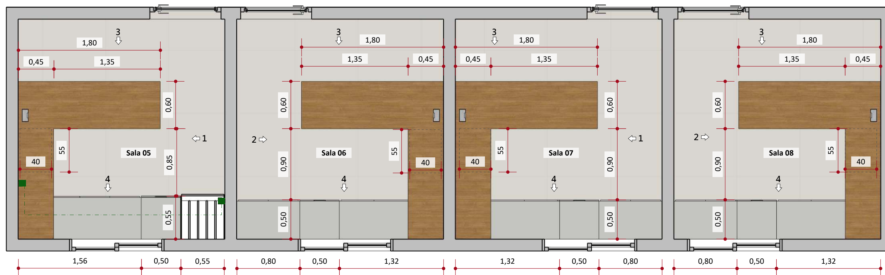
Planta Marcenaria ESCALA 1:30
