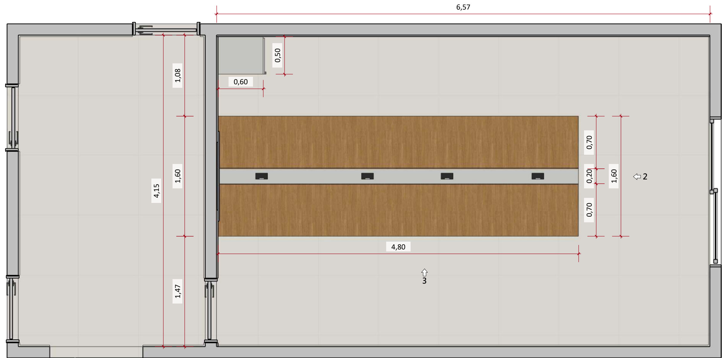
Planta Marcenaria ESCALA 1:30
