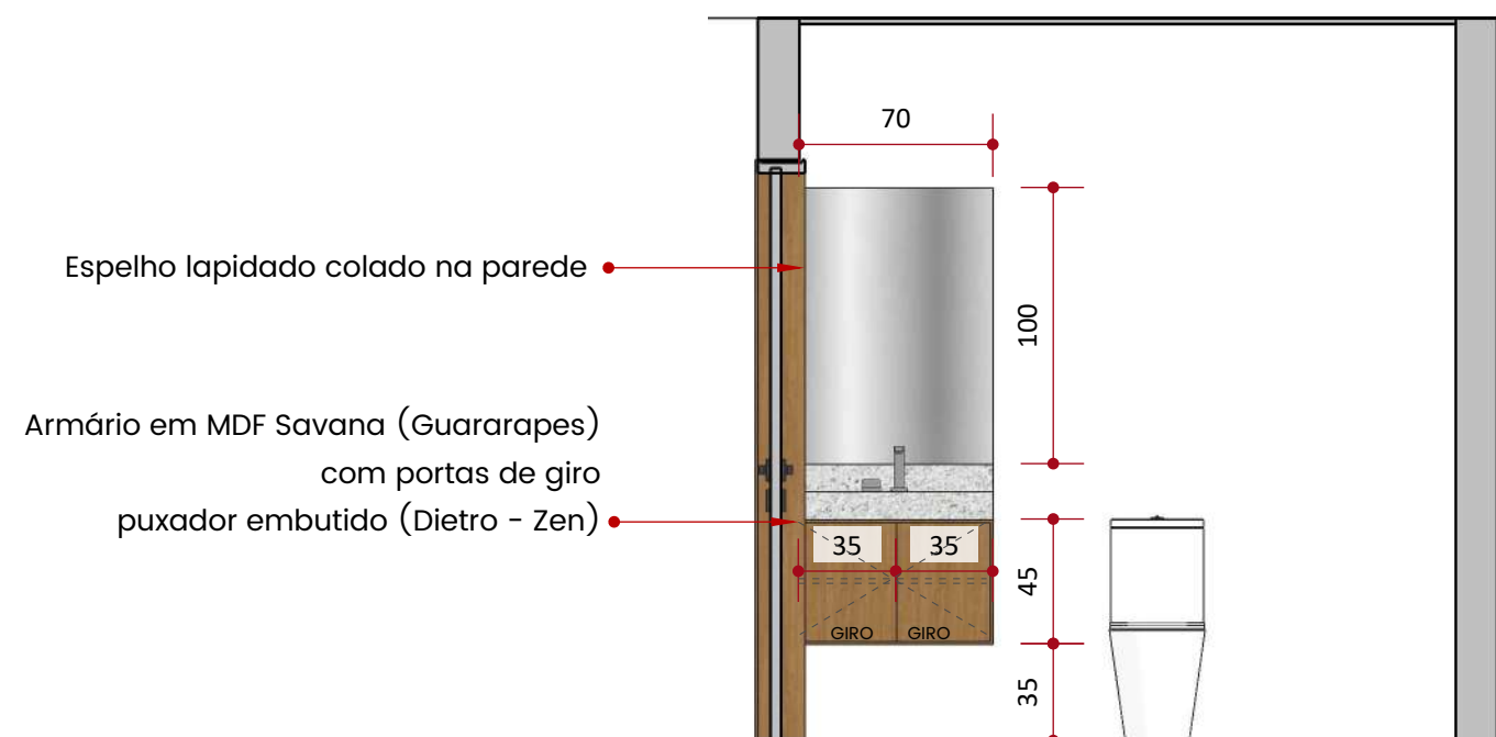
Vista 06 ESCALA 1:30
