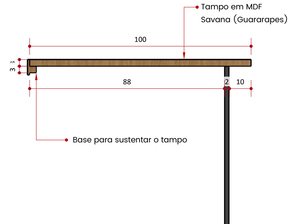
VISTA LATERAL
