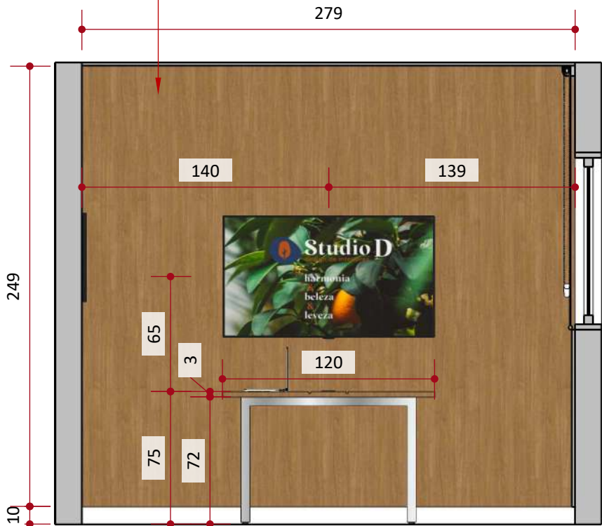
Vista 2 ESCALA 1:30
