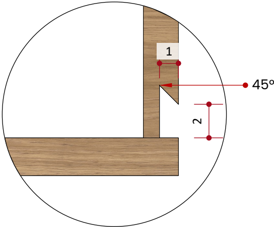
Detalhe Puxador Cava S/Escala
