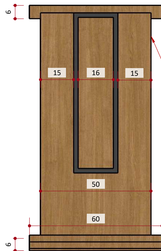
VISTA SUPERIOR MESA FECHADA
