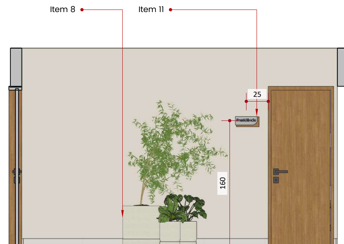
Vista 4 - Corredor ESCALA 1:30
