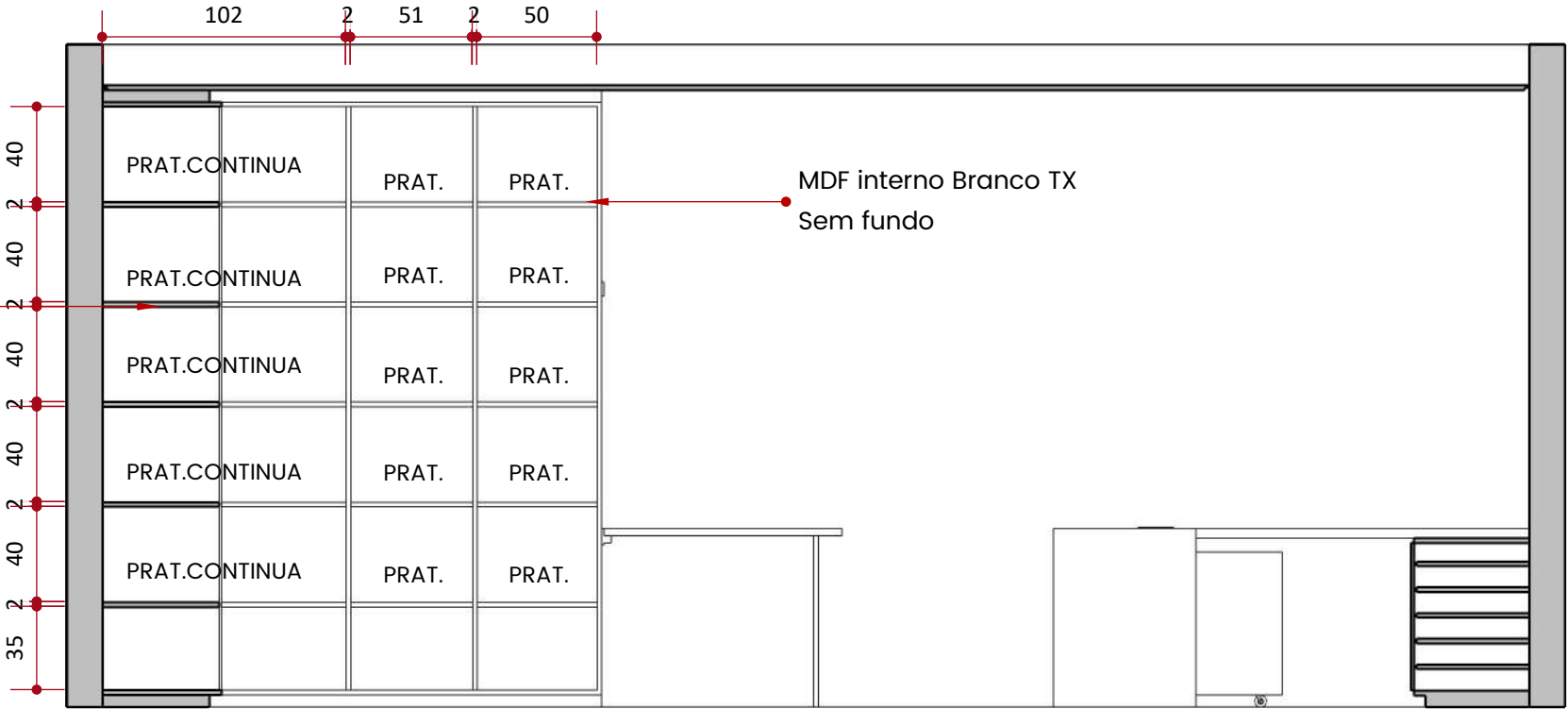
Vista 03 - Interno ESCALA 1:30
