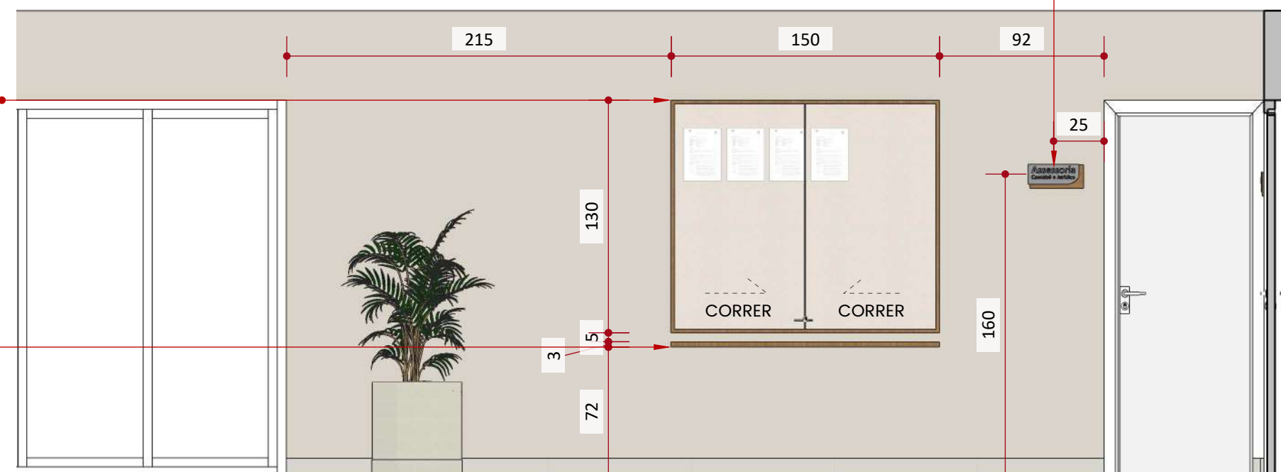
Vista 3 ESCALA 1:30
