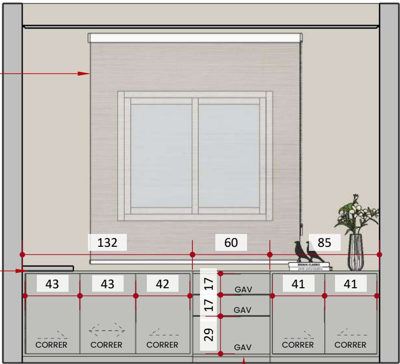
Vista 5 ESCALA 1:30
