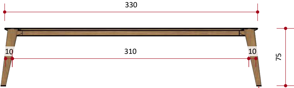
VISTA LATERAL
