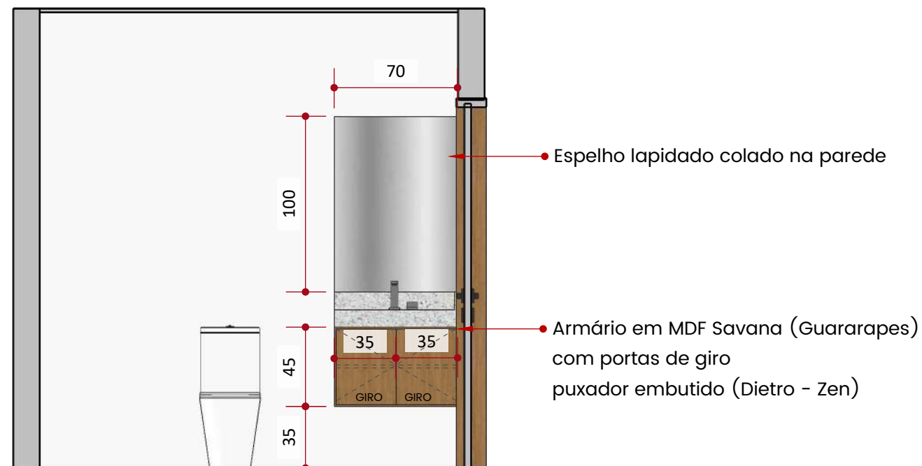
Vista 5 ESCALA 1:30
